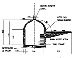
SECCIÓN A - A
